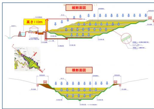
管理型最終処分場の概念図（２）
